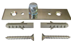
Pivot Plate TK 9124
